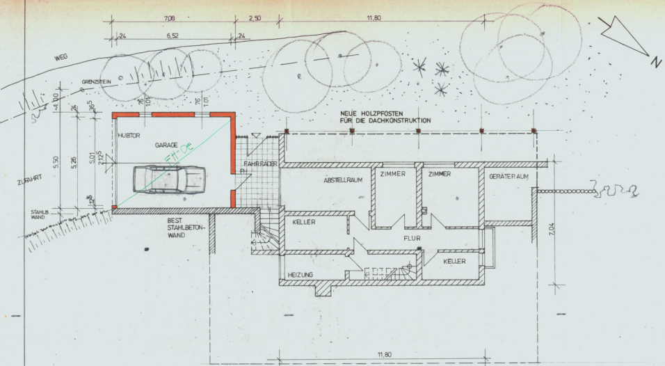
KELLERGESCHOSS NEUE GARAGE
