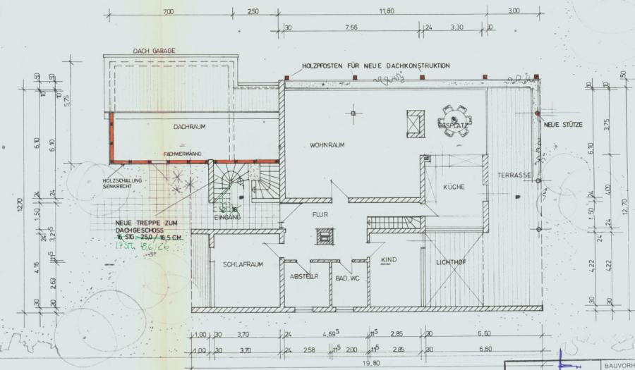
ERDGESCHOSS NEUE GARAGE
